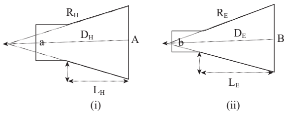
Fig. 4. (i) H-plane (ii) E-plane of the pyramidal horn antenna.
